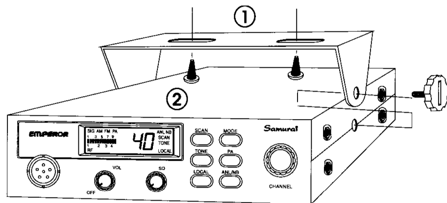
SCHÉMA GÉNÉRAL DE MONTAGE
